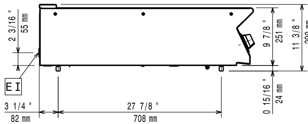
侧视
